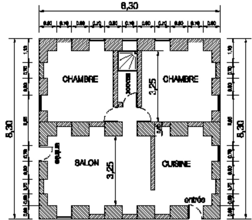
MAISON STANDART pour une famille (deux chambres, salon, douche, cuisine) +/- 55 m 2
