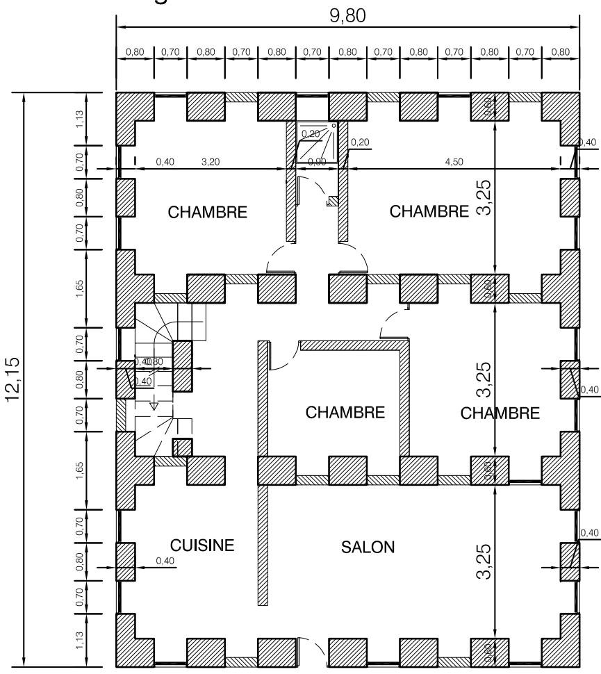
MAISON A ETAGE rez de chaussée
