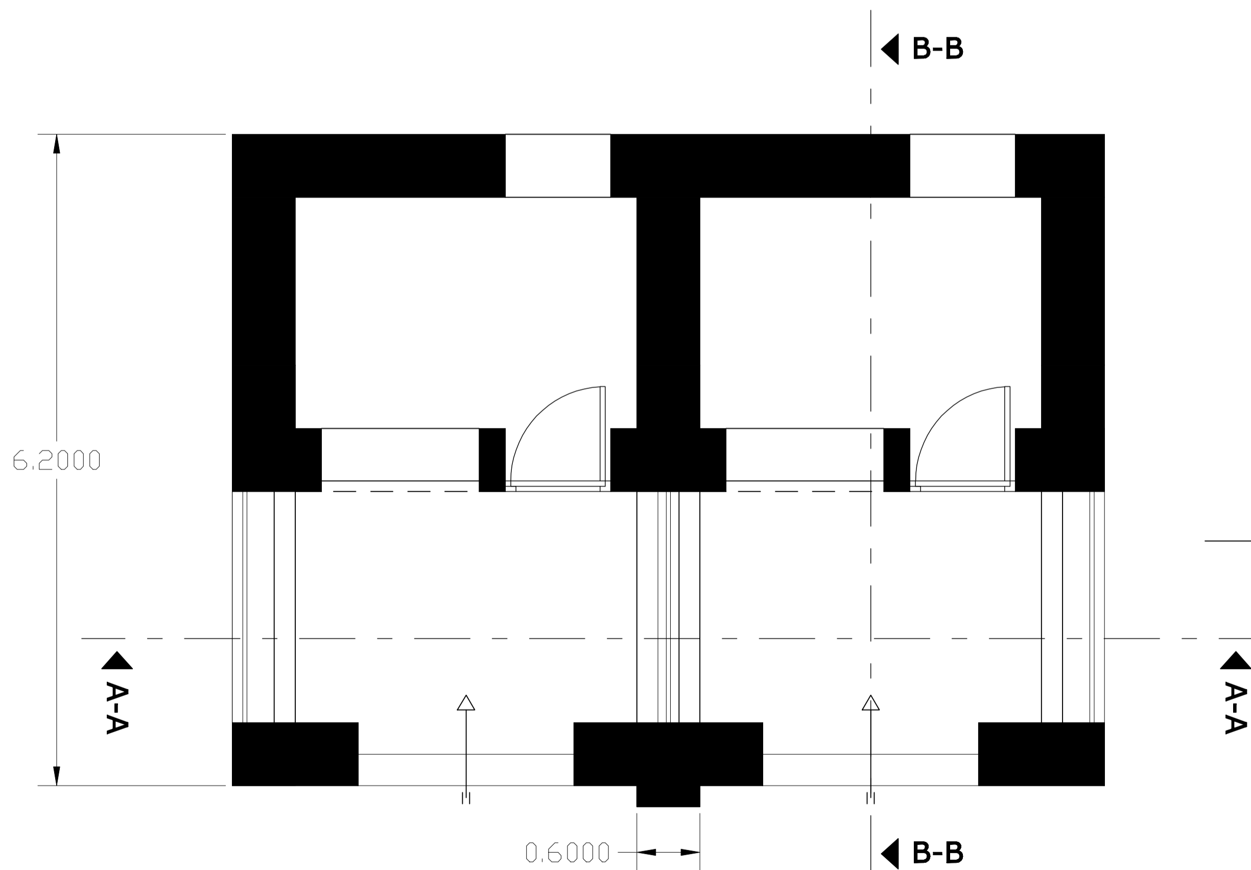
Plan Niveau
