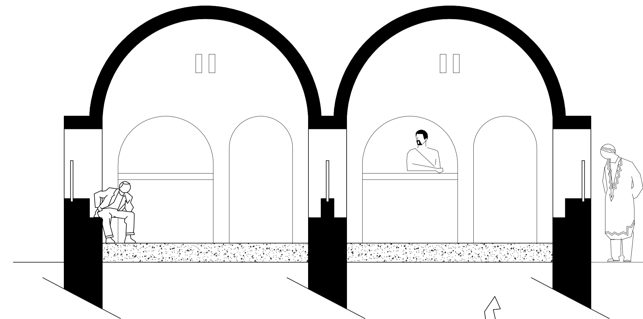
Coupe A-A
