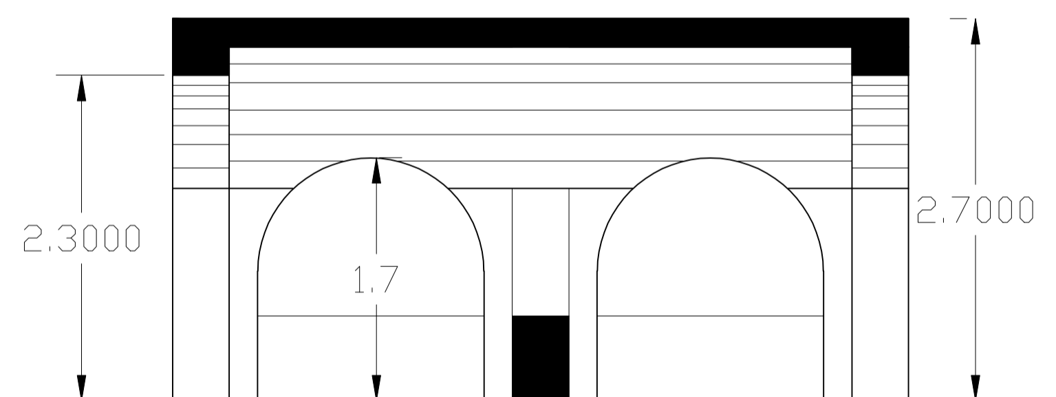
Coupe B-B
