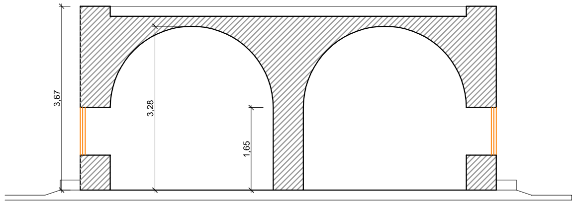
COUPE A-A
